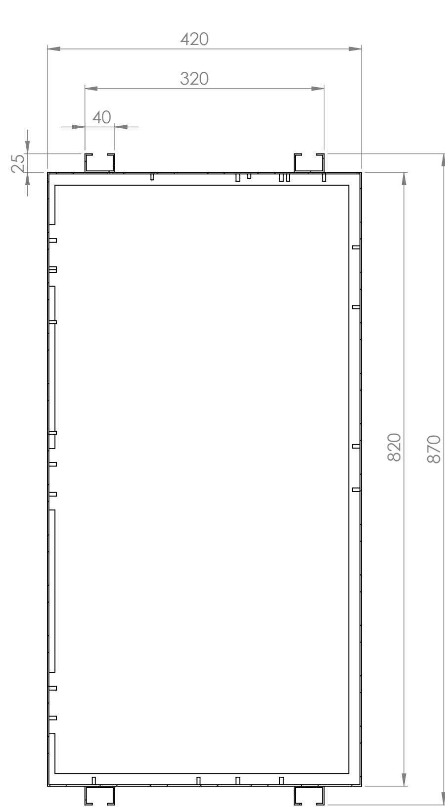
COUPE A-A ECHELLE 1 : 5
